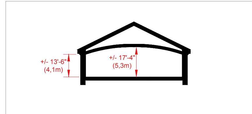
Dégagement / Clearance
