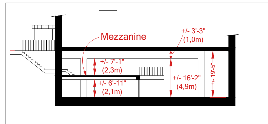
Dégagement / Clearance
